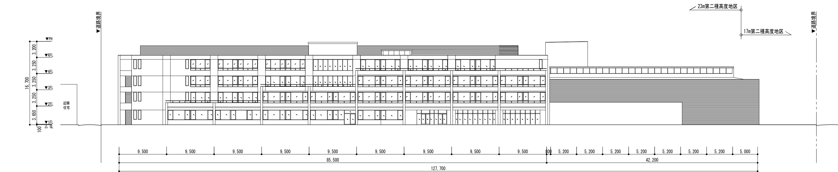
北立面图 S=1/400
