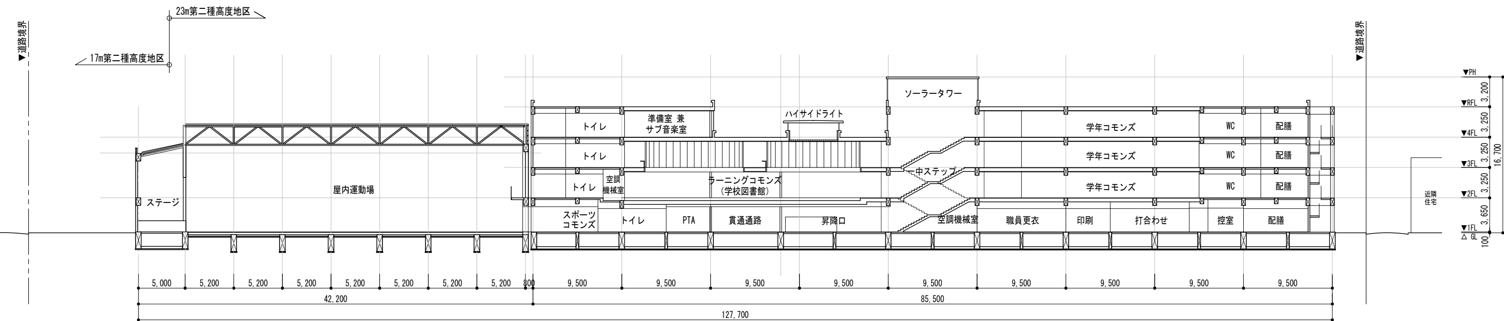
A-A断面図 S=1/400
