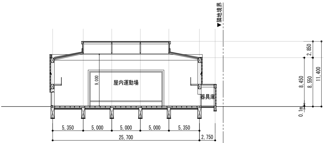
C-C断面図 S=1/400
