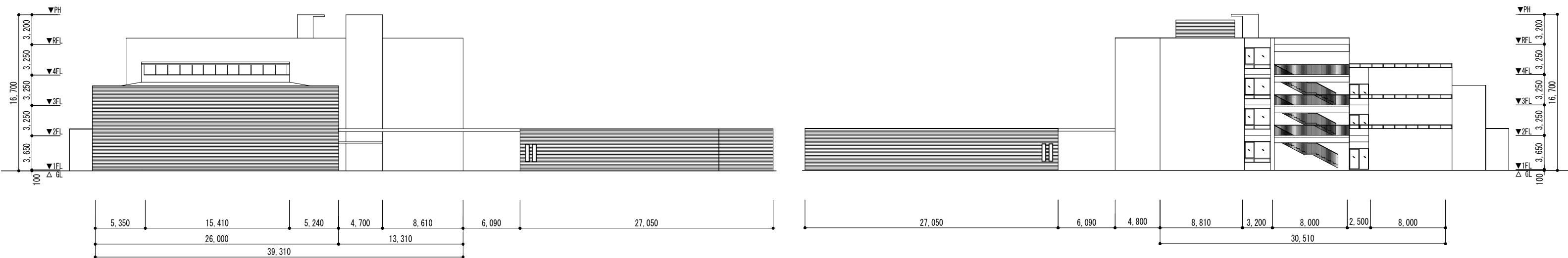
西立面图 S=1/400
