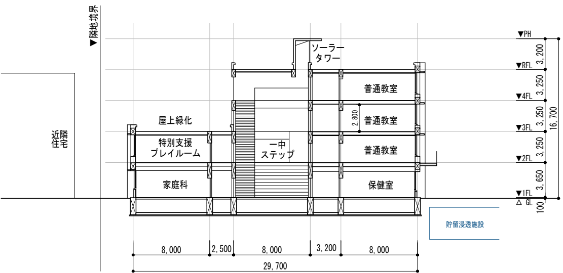
B-B断面図 S=1/400
