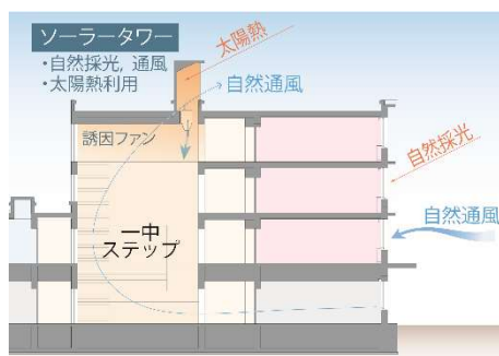
ソーラータワーイメージ（一中ステップ断面）
