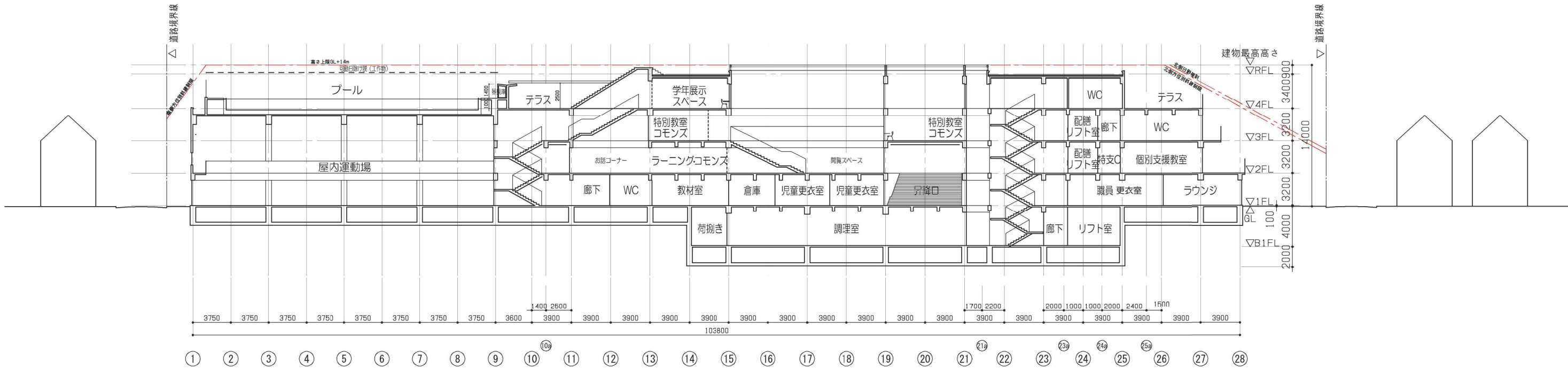
A-A' 断面図
