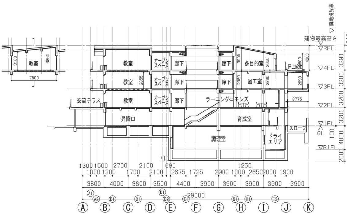
B-B' 断面図
