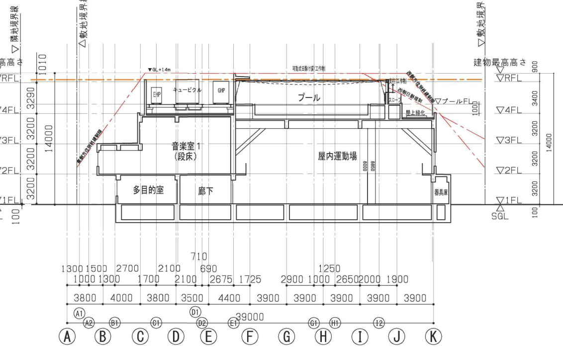
D-D' 断面図
