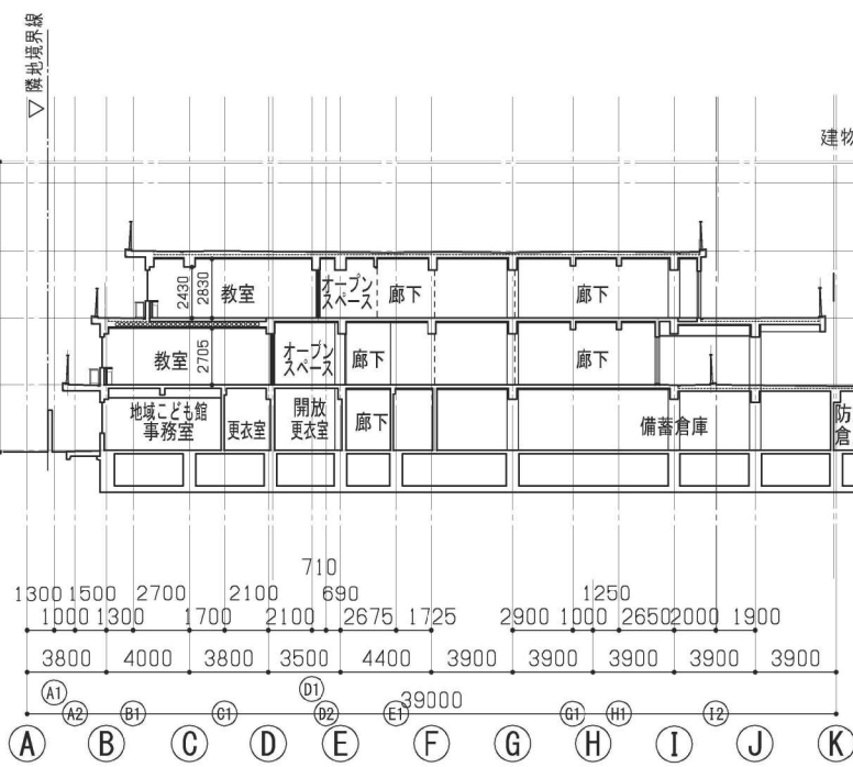
C-C' 断面図
