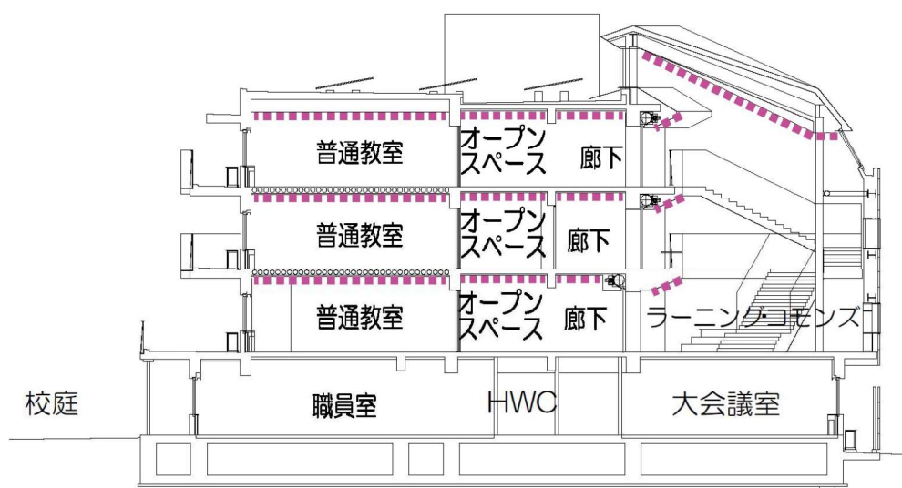
吹抜けの断面形状と音環境の図
