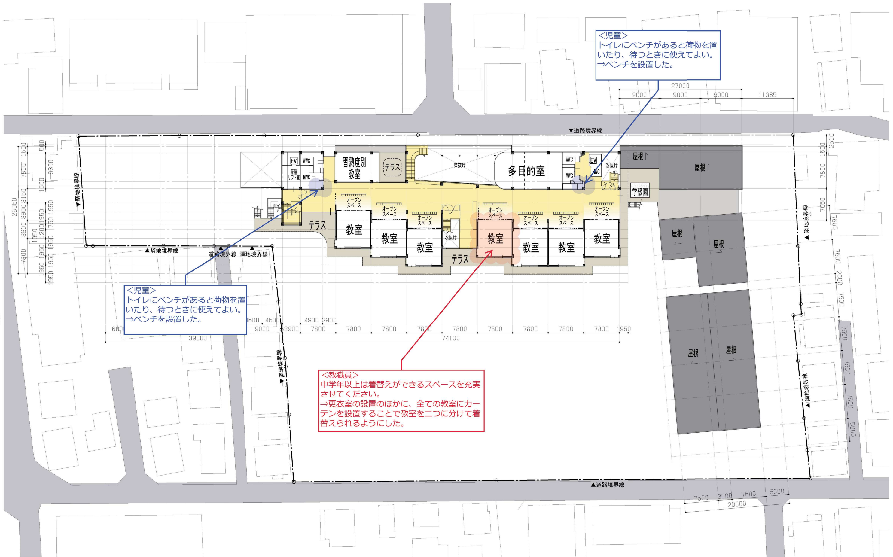
武蔵野市立第五小学校 4階平面図
