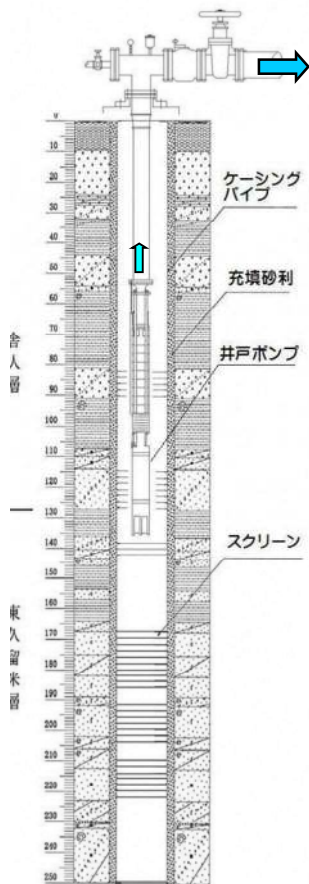
柱状図
